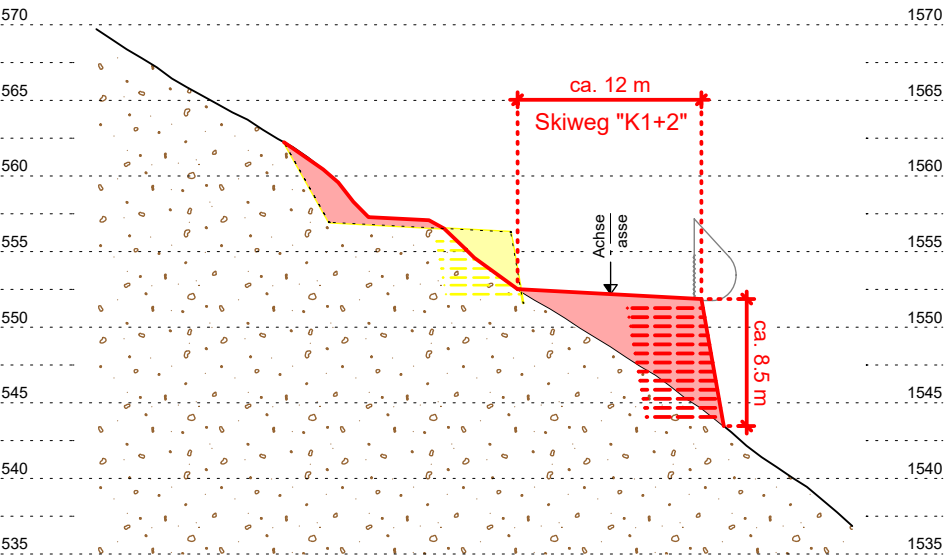
QUERSCHNITT / SEZIONE TRASVERSALE K25bis Mst./Sc. 1:500
