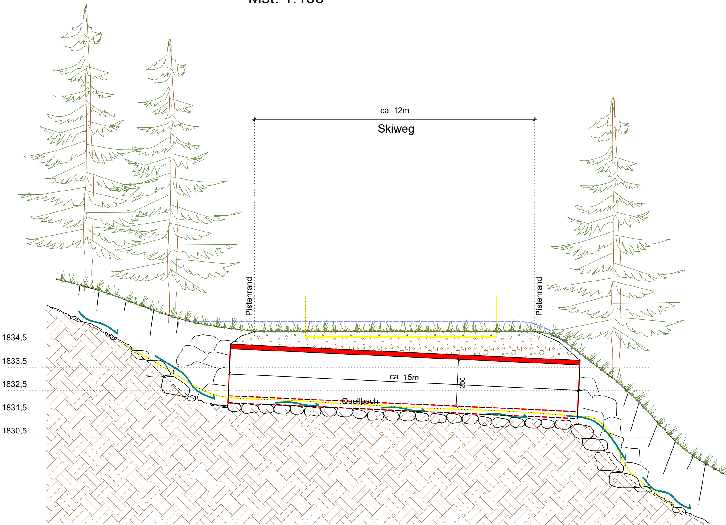
SCHNITT L1-L1 Mst. 1:100
