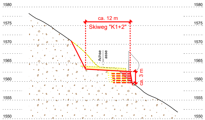
QUERSCHNITT / SEZIONE TRASVERSALE K23bis Mst./Sc. 1:500
