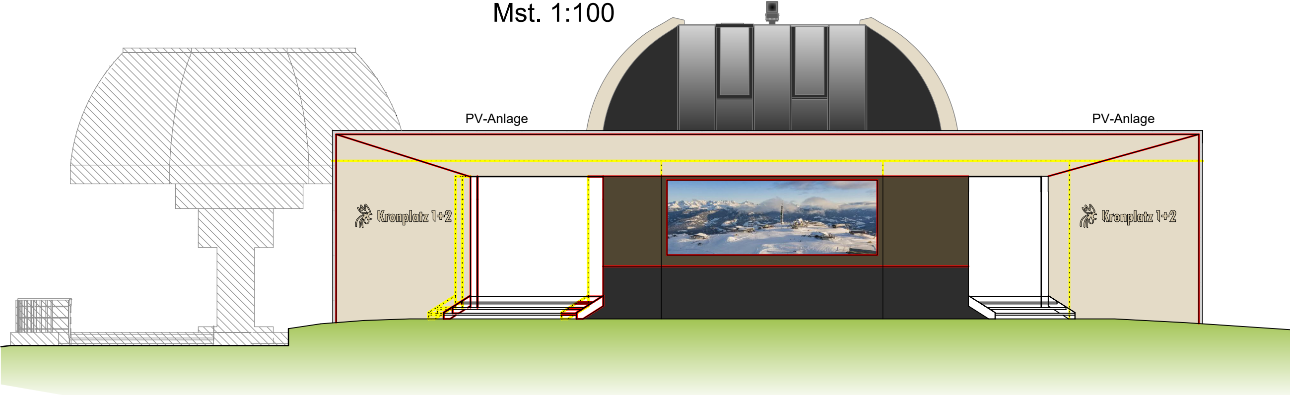
SÜDANSICHT Mst. 1:100
