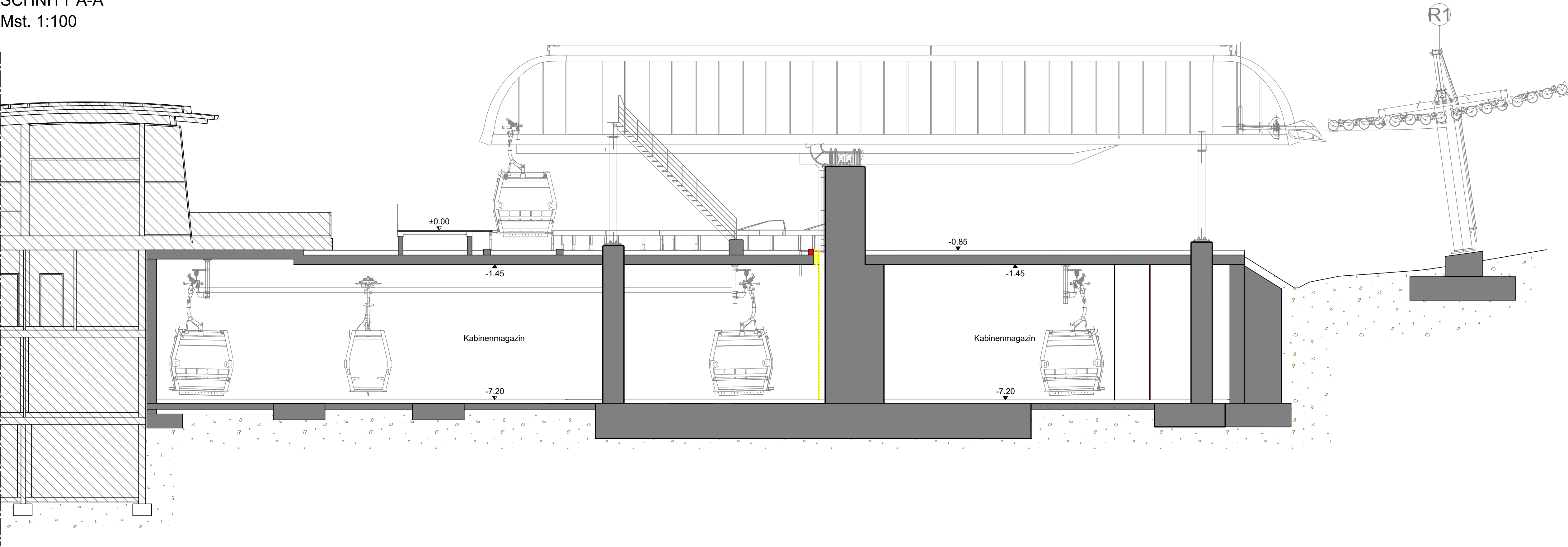
SCHNITT B-B Mst. 1:100
