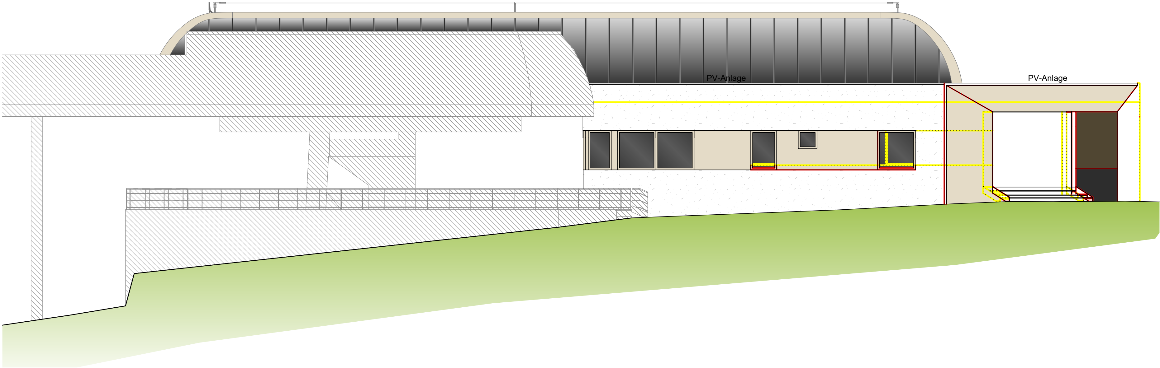
WESTANSICHT Mst. 1:100
