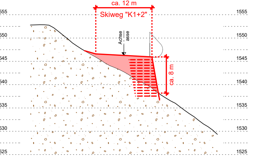
QUERSCHNITT / SEZIONE TRASVERSALE K26 Mst./Sc. 1:500
