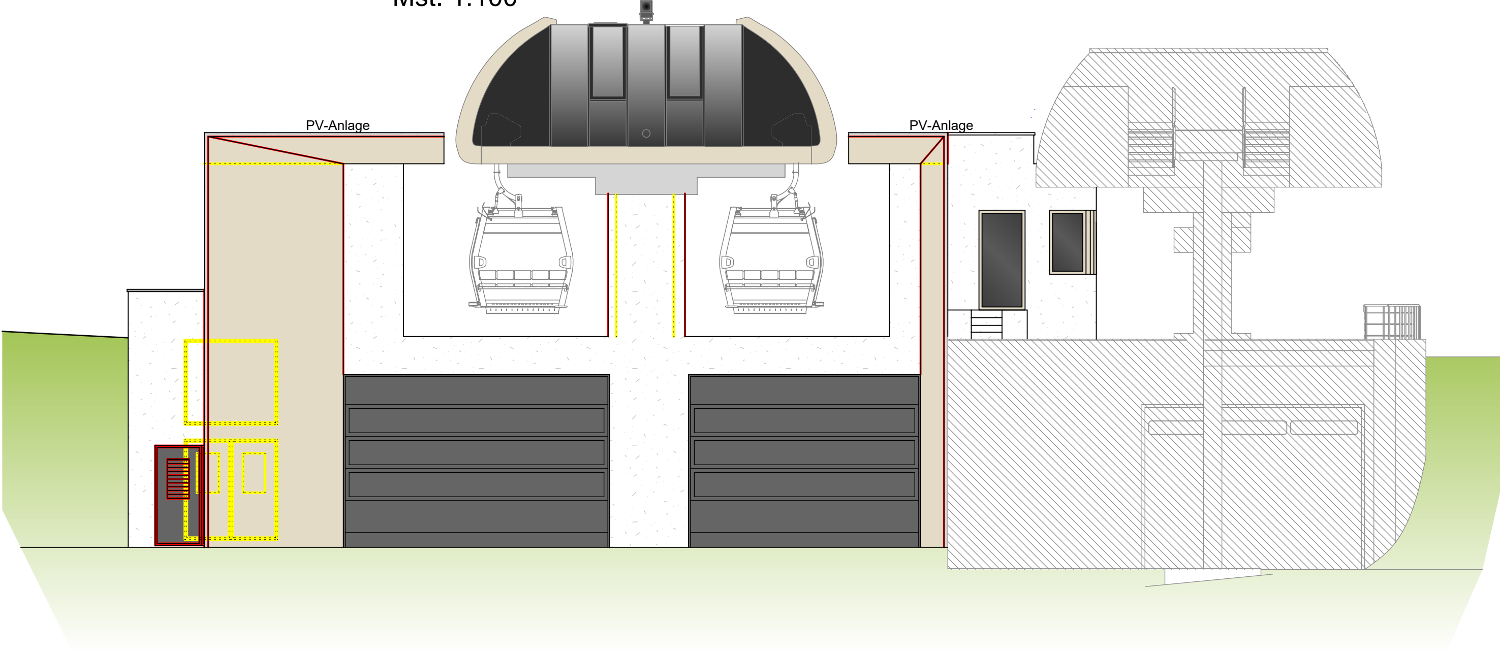
NORDANSICHT Mst. 1:100
