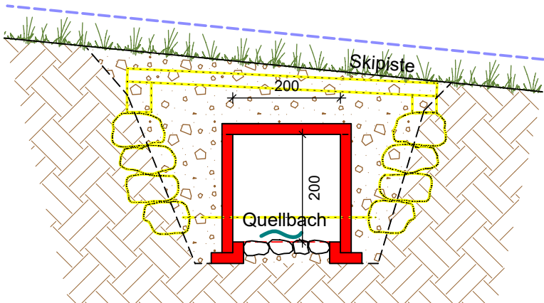
SCHNITT Q1-Q1 Mst. 1:100
