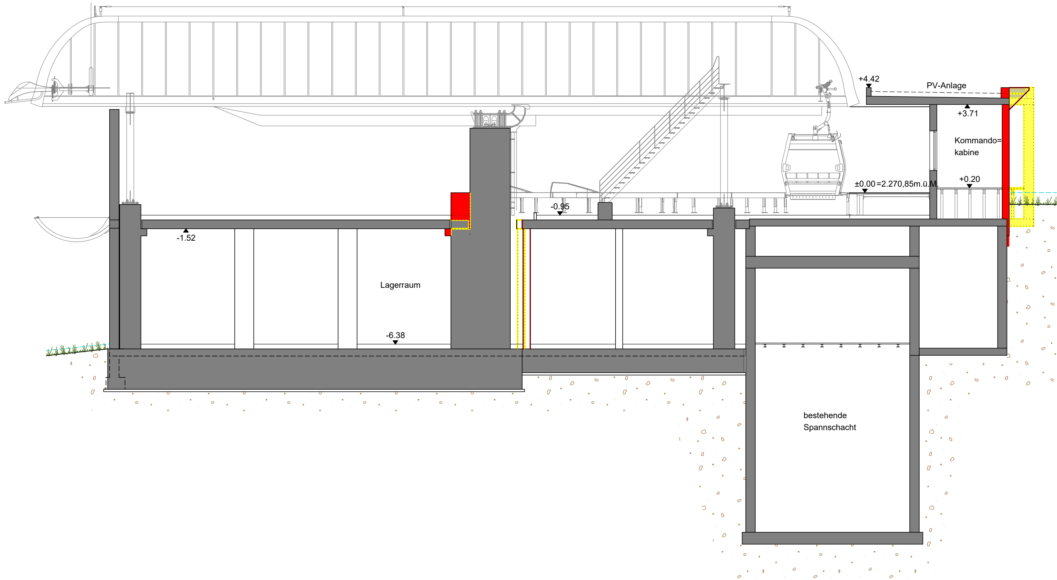
SCHNITT A-A Mst. 1:100
