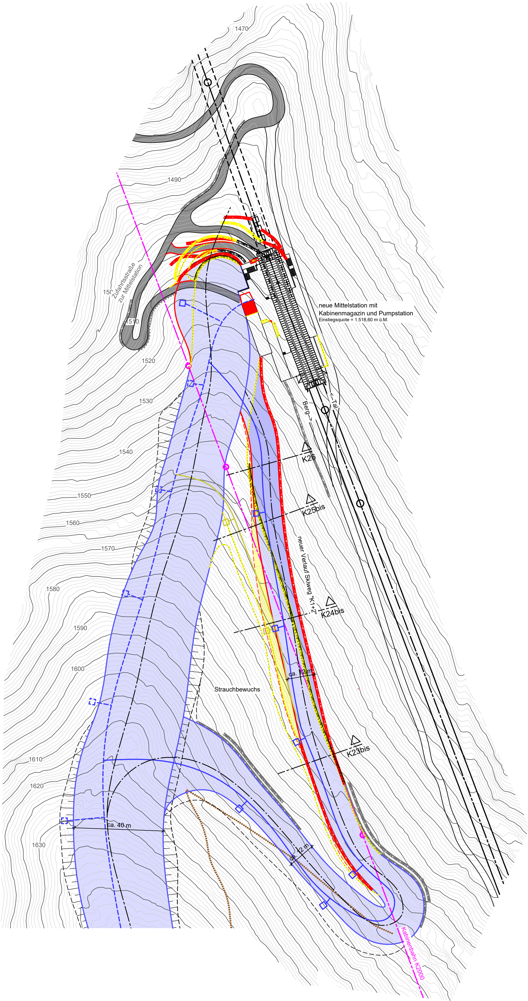
LAGEPLAN SKIPISTE UND SKIWEG "K1+2" Mst. 1:1.000
