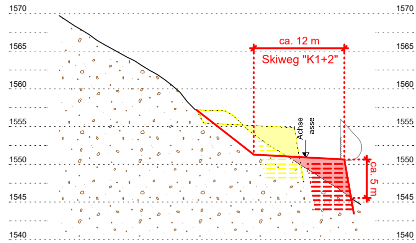
QUERSCHNITT / SEZIONE TRASVERSALE K24bis Mst./Sc. 1:500
