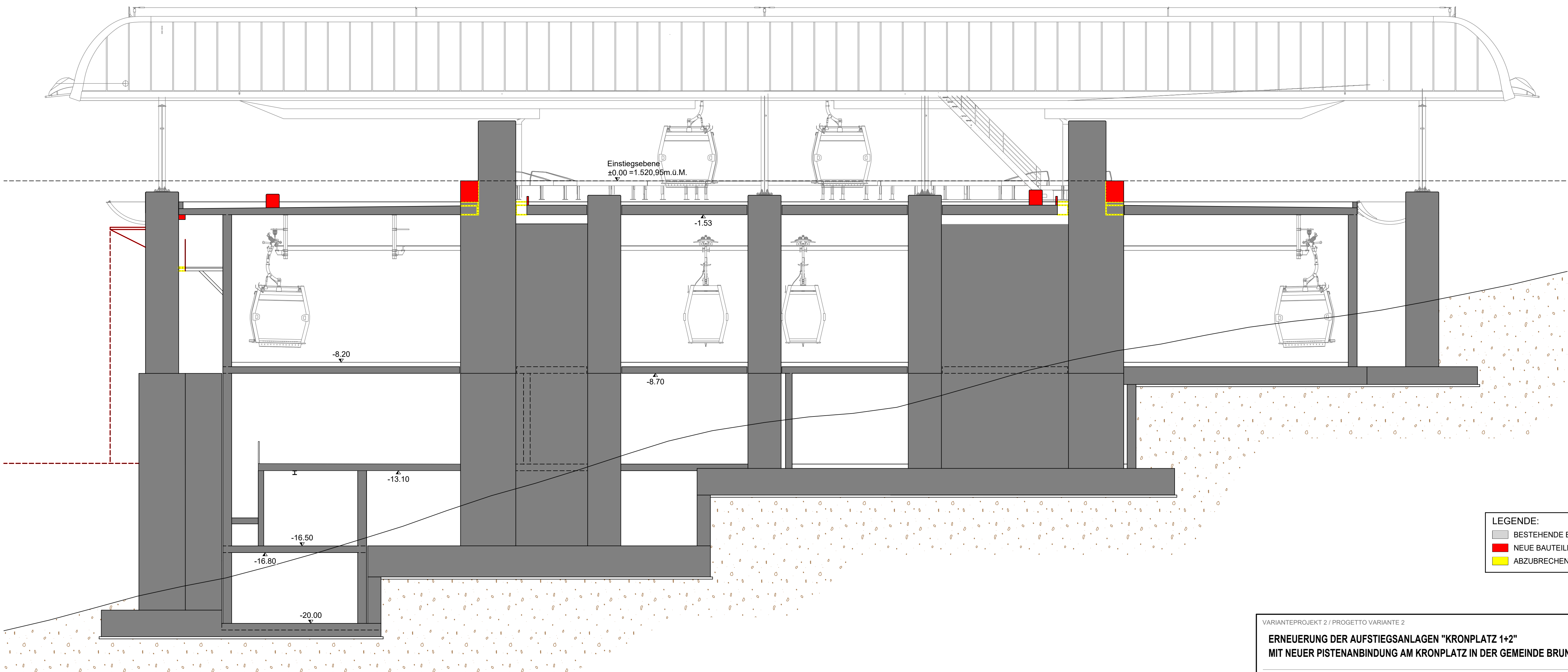
SCHNITT A-A Mst. 1:100
