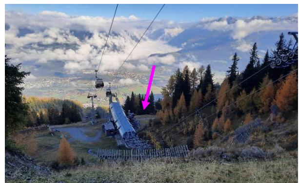
Übersichtsfoto der bestehenden Mittelstation mit Position der geplanten Stütze II-06 „Kronplatz 2“
