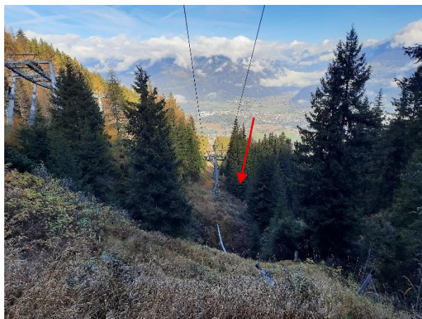
Übersichtsfoto der Baufläche von Stütze II-04
