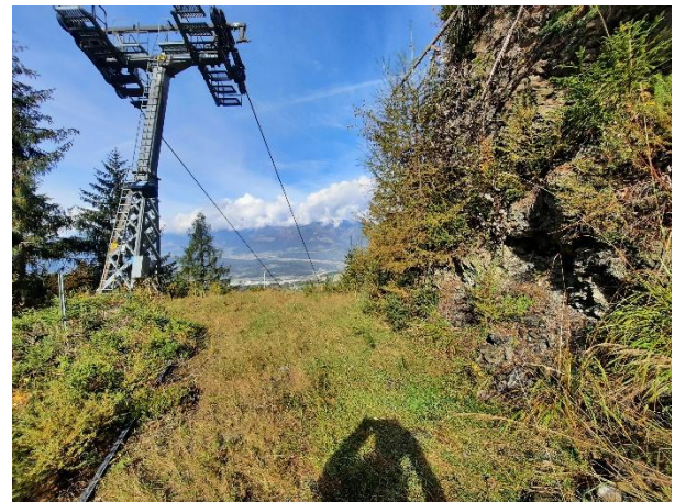
Bestehende Stütze 13 knapp talseitig der geplanten Stütze I-08
